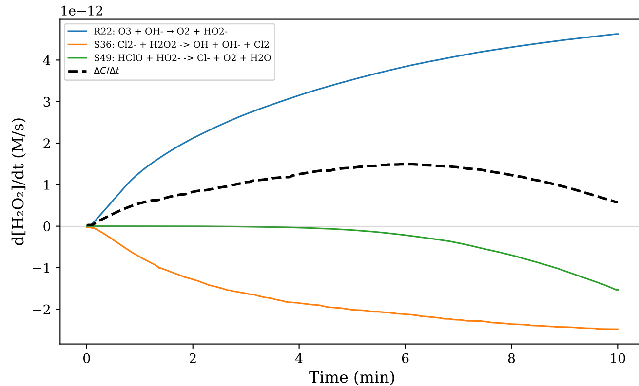
(d) \text{H}_2\text{O}_2
